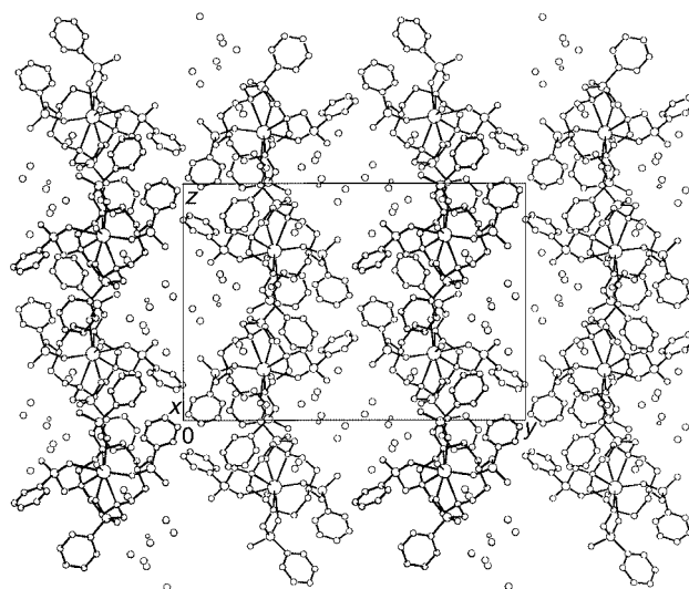
Fig. 4 Crystal packing of Li[La(L 1 )(H 2 O)]·10H 2 O.
